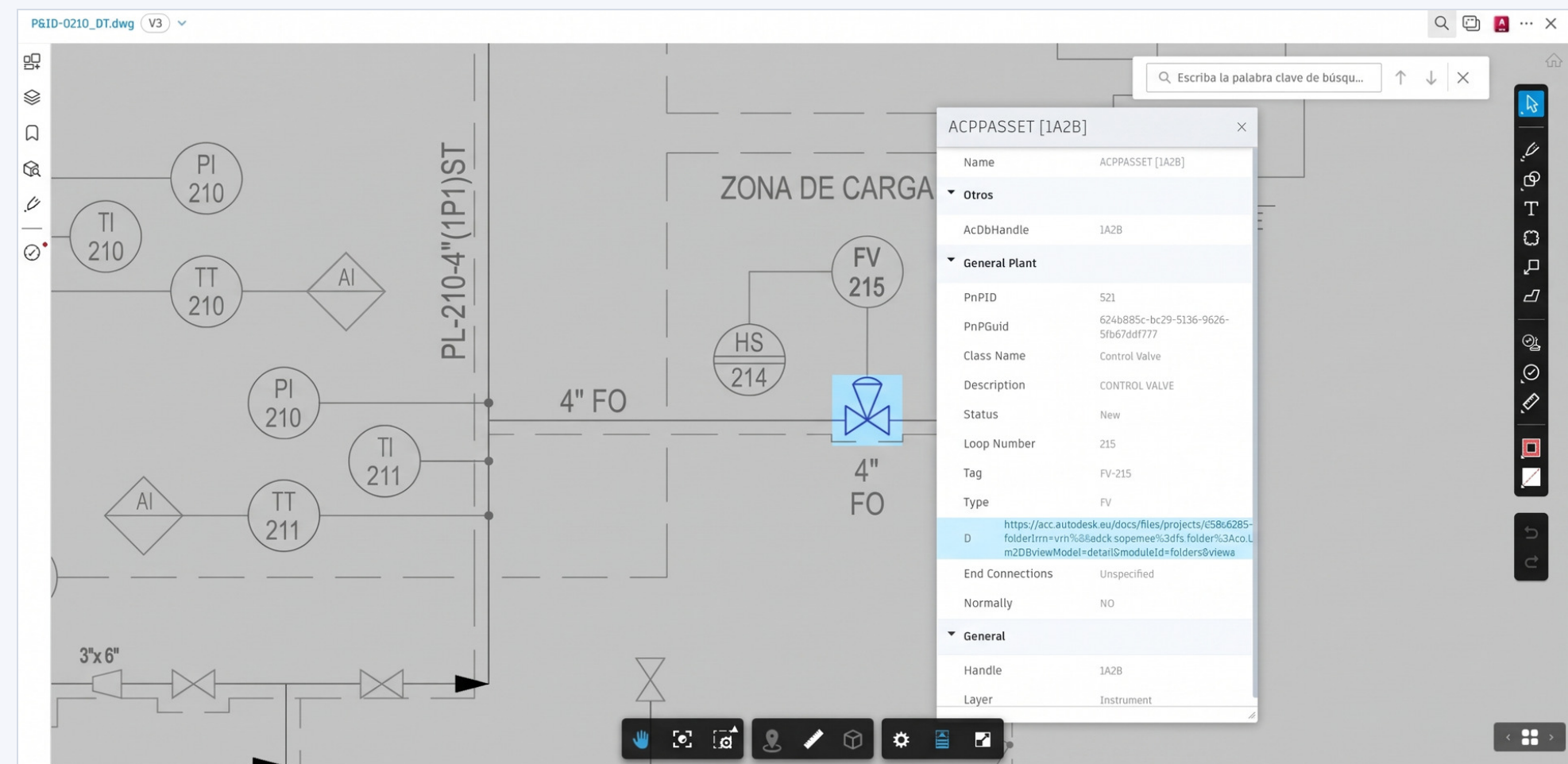
Un P&ID inteligente: al seleccionar una válvula se despliegan sus propiedades. Esquema y códigos de demostración.
